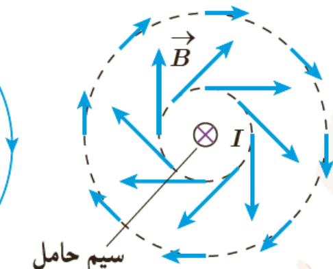
سیم حامل جریان درون سو
